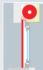
Pose dans coffre existant enroulement intérieur
